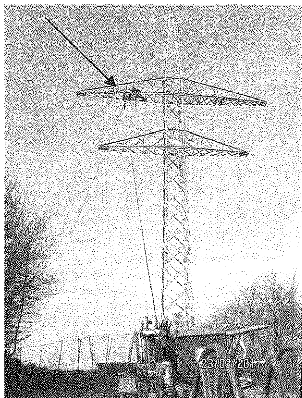
Abb.2: In schwindelnder Höhe wird von einem Monteur auf dem Abspannmast im Rautal ein Laufrad angebracht (Pfeil).
