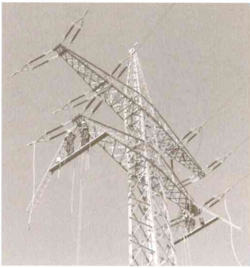
Abb. 4: In etwa 20m Höhe werden von schwankenden Arbeitsbühnen aus die 6 Leiterseilenden zweier Zugabschnitte über eine Stromschleife verbunden.
