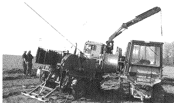
Abb. 3: „Abwickelstelle“ am Ziskauer Tal. Das Leiterseil wird von der neuen Seilrolle abgezogen.
