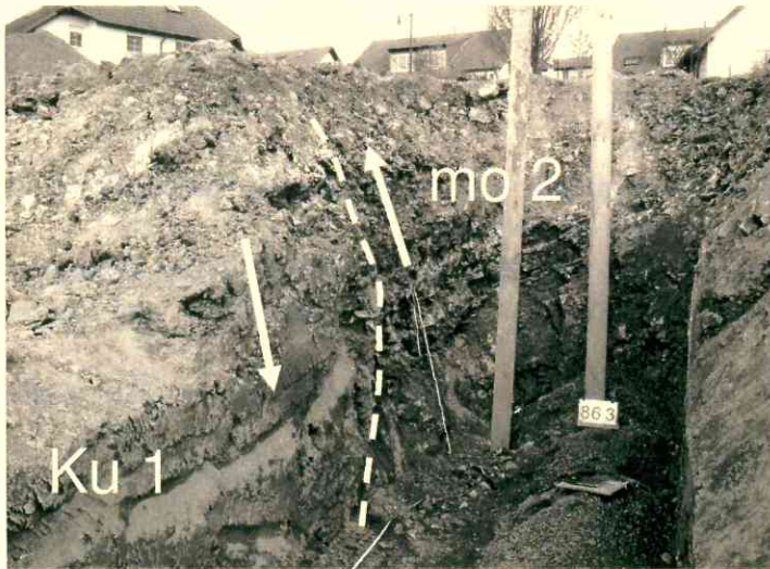
Abb. 2: Erster Hausanschluss südlich des Starweges. Die östliche Grabenstörung zwischen dem Unteren Keuper (ku 1) und dem Oberen Muschelkalk (mo2) ist durch die gerissene Linie markiert.
